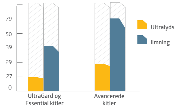
Ærmesømmenes gennemsnitlige strækstyrke (N)
